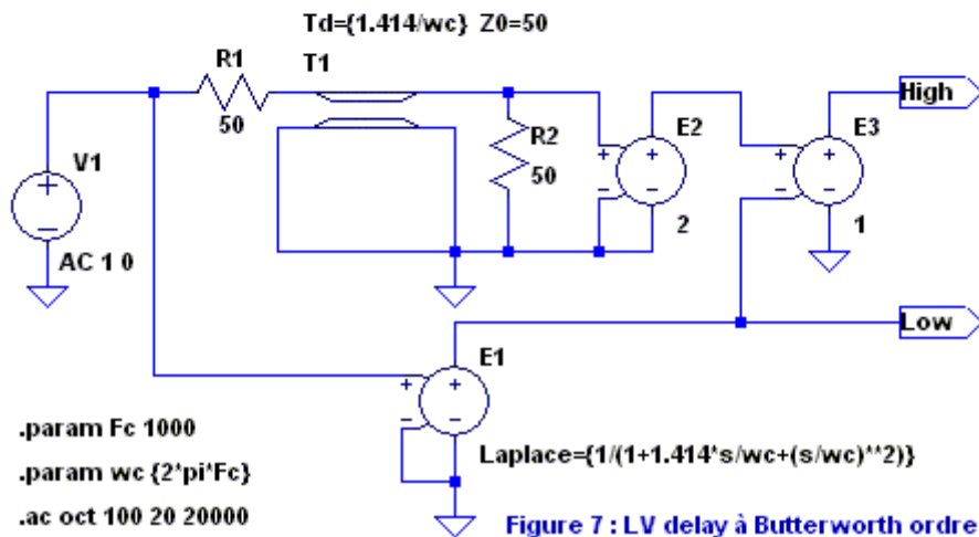
Figure 7 : LV delay à Butterworth ordre 2
