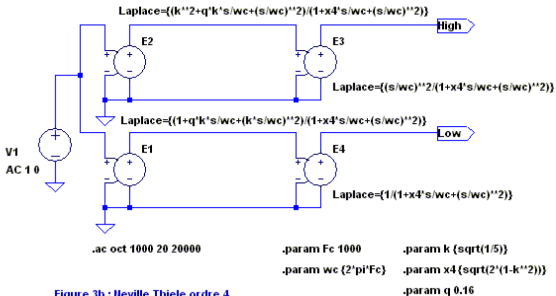
Figure 3b : Neville Thiele ordre 4
