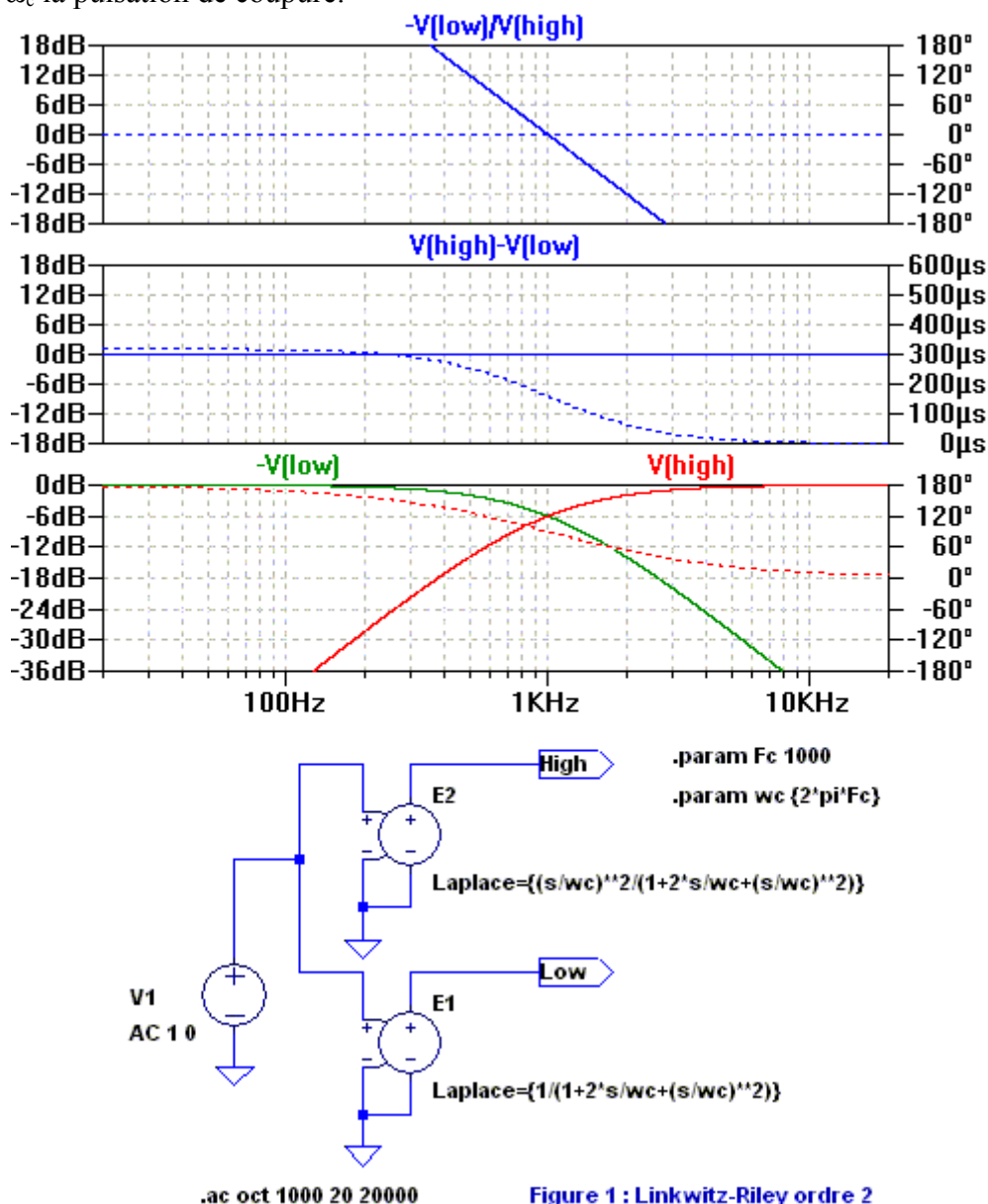
Figure 1 : Linkwitz-Riley ordre 2
